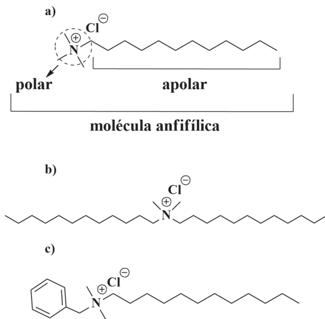
Figura 5. Exemplos de surfactantes catiônicos. Cloreto de (a) dodeciltrimetilamônio, (b) didodecildimetilamônio e (c) dodecilbenzildimetilamônio
