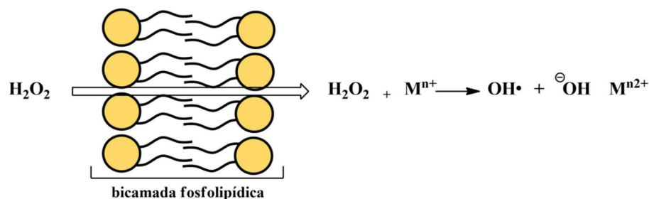
Figura 7. Representação da entrada do peróxido de hidrogênio através da membrana e posterior formação do radical \text{OH}\cdot
